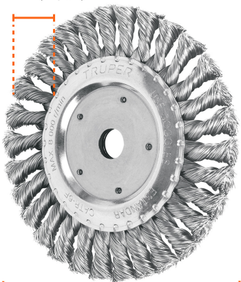
Diámetro 6" (150 mm)
