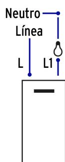
Interruptor sencillo
