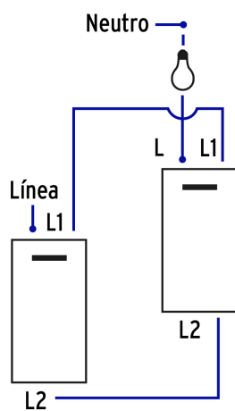
Interruptor 3 vías
