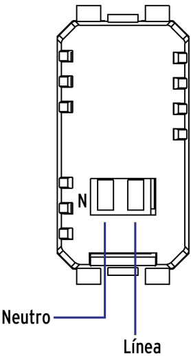
Diagrama de conexión
