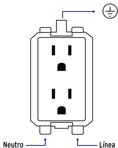
Diagrama de conexión
