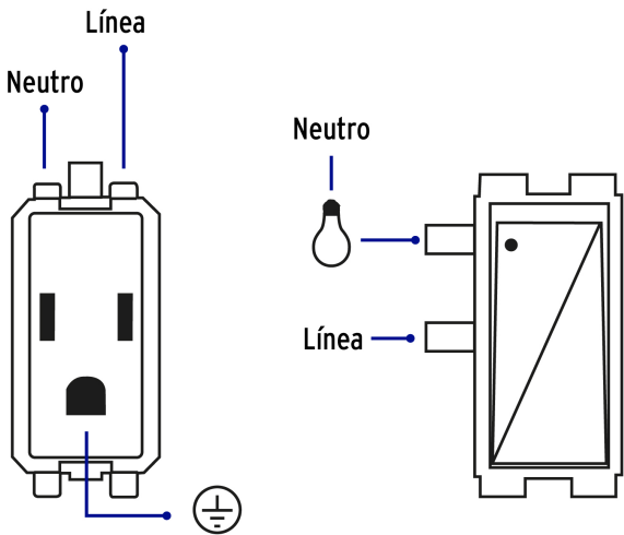
Diagrama de conexión
