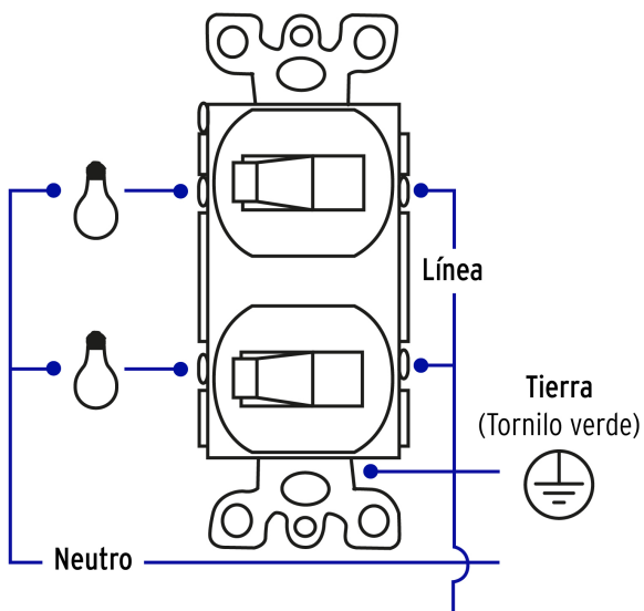
Diagrama de conexión
