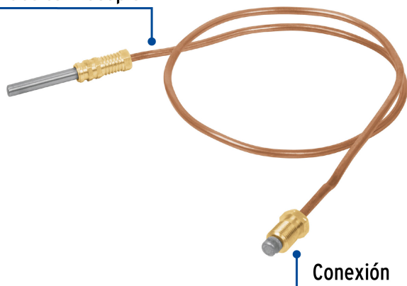
Tubo termocople
