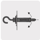
Taquete montado
